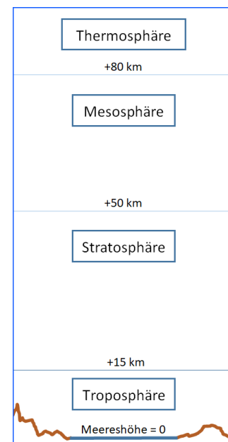
Bild 2: Aufbau untere Atmosphäre
