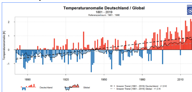
Bild 13: Temperaturanomalie Deutschland / Global (Quelle DWD) [19]
