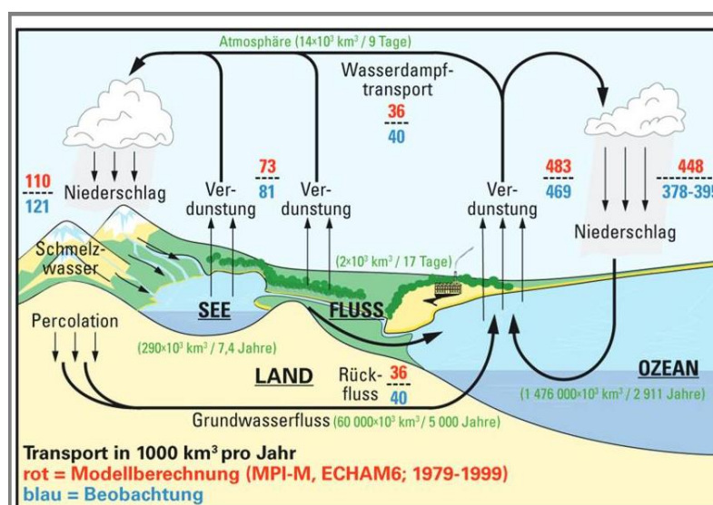
Bild 9: Globaler Wasserkreislauf [14]
