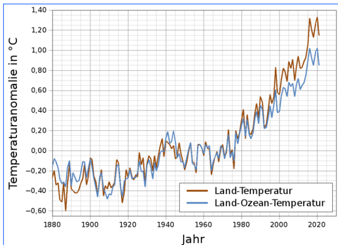
Bild 14: Mittlere Temperaturanomalie Land/Wasser [20]
