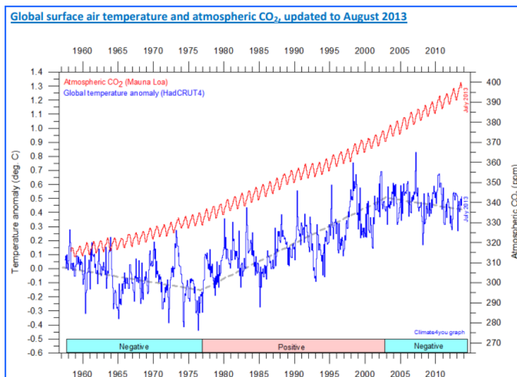
Bild 7: Globale Temperaturschwankungen [11]
